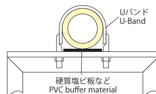
硬質塩ビ板など PVC buffer material <参考> Uバンドによる固定支持 <Note> Fixed support from u-band
