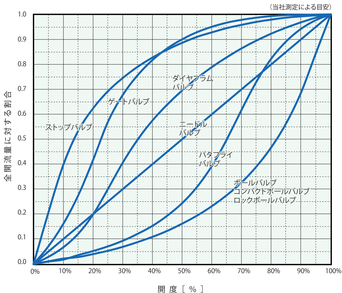
エスロンバルブの開度と流量の関係
