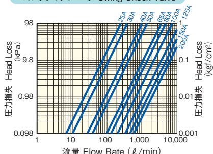
スイングチャッキバルブ Swing Check Valve
