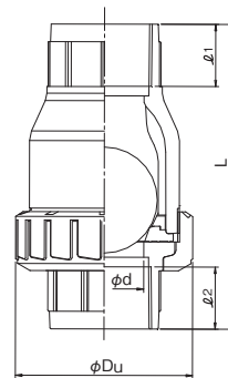
●ねじ式 Thread Type
