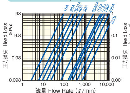
ダイヤフラムバルブ Diaphragm Valve
