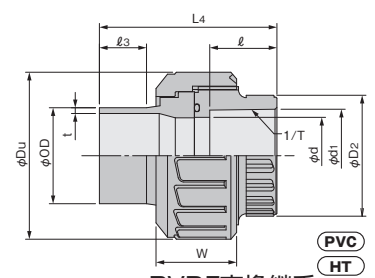
PVDF変換継手 PVDF Transtion (TS Socket-Butt)
