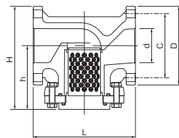
●フランジ式 Flange Type (65~100A)
