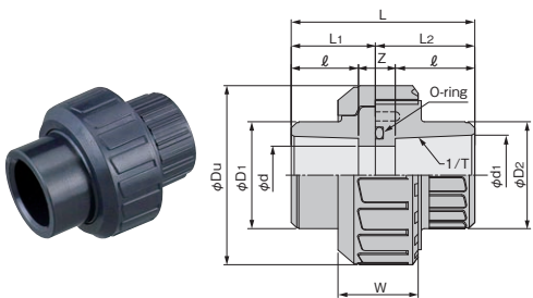
PVC, HT(C-PVC) リング O-ring :EPDM or FKM
