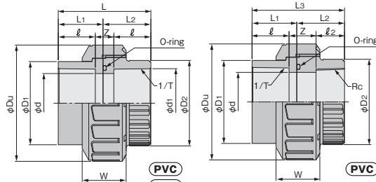
TSソケット TS Socket
