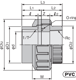
ねじ変換継手 Thread Transtion (TS Socket-Thread)
