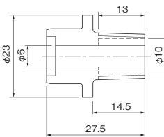
●ホース受口 Hose
