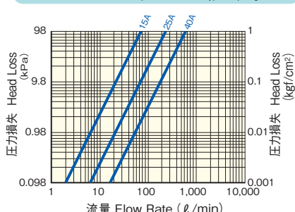
分岐ダイヤフラムバルブ Dead Space Free Tee-Type Diaphragm Valve
